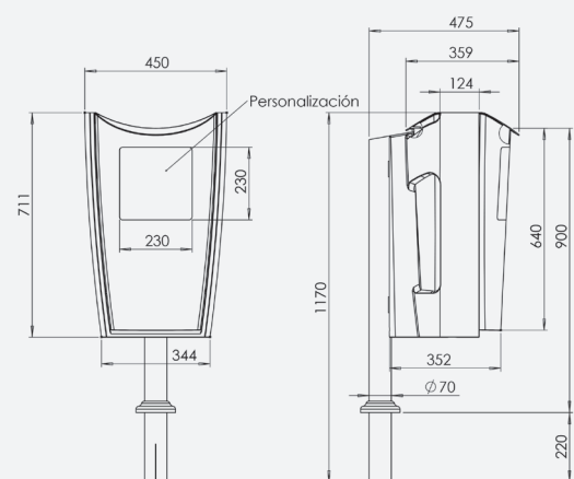
PAPELERA OMEGA 50 L DESCUBIERTA
